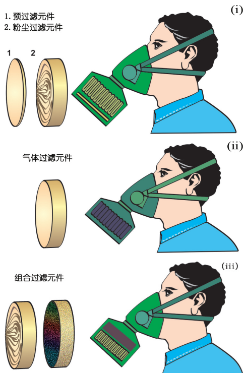
图102a (i) (ii) (iii) 显示了三种有过滤元件的半面罩呼吸防护罩类型。
